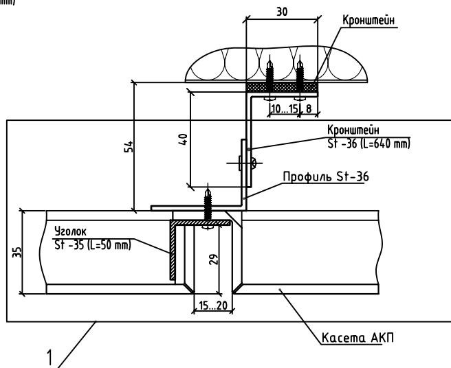
Схема установки кассет
